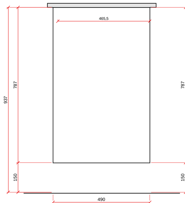
VISTA C - ESC. 1:10
