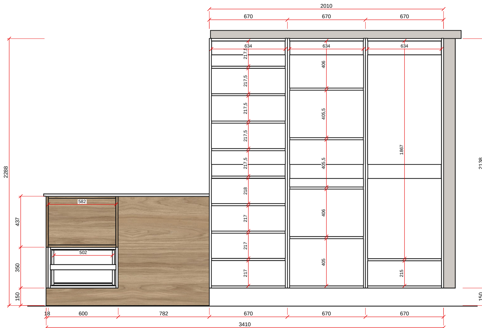
VISTA B - ESC. 1:20
